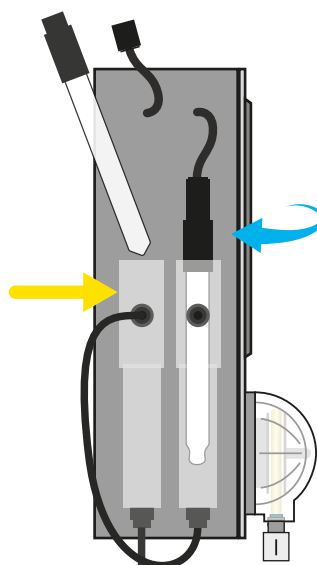
Sondendurchflussarmatur für die CLF-Sonde oder die Redox-Sonde
